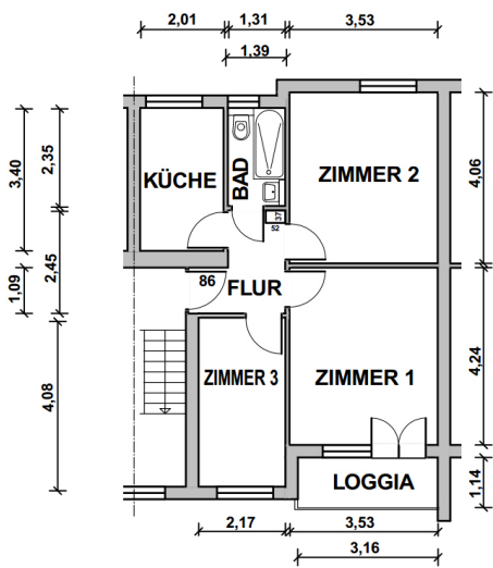
Grundriss
